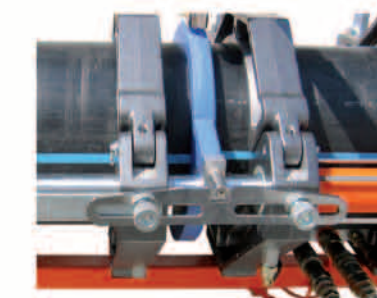
Фиксация нагревателя
